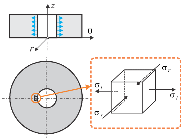
Фиг. 10. Напрегнато състояние по време на студено разширение за методите от подгрупа A.1.2
