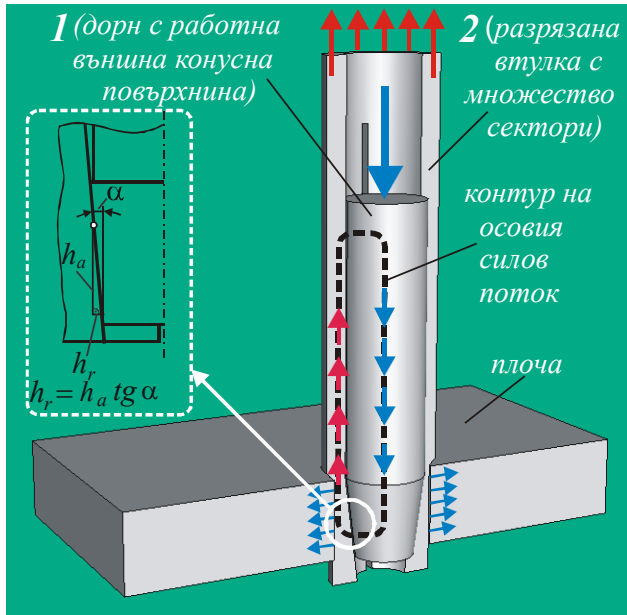
Фиг. 9. Принципно схем на метод за чисто радиално разширение посредством множество радиално подвижни сектори
