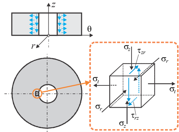
Фиг. 7. Напрегнато състояние за методите от подгрупа А.1.1 по време на студено разширение
