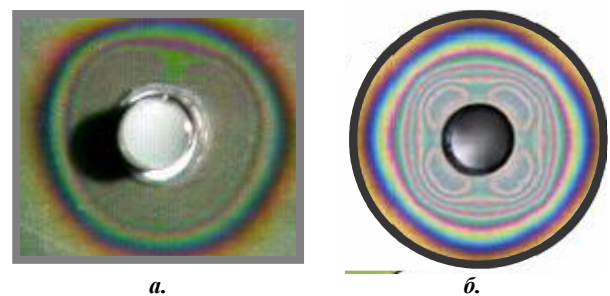
Фиг. 8. Разпределение на зоната с \sigma_t^{res} в окръжно направление а. при метода Split Sleeve Cold Expansion; б. при метода Slit Mandrel
